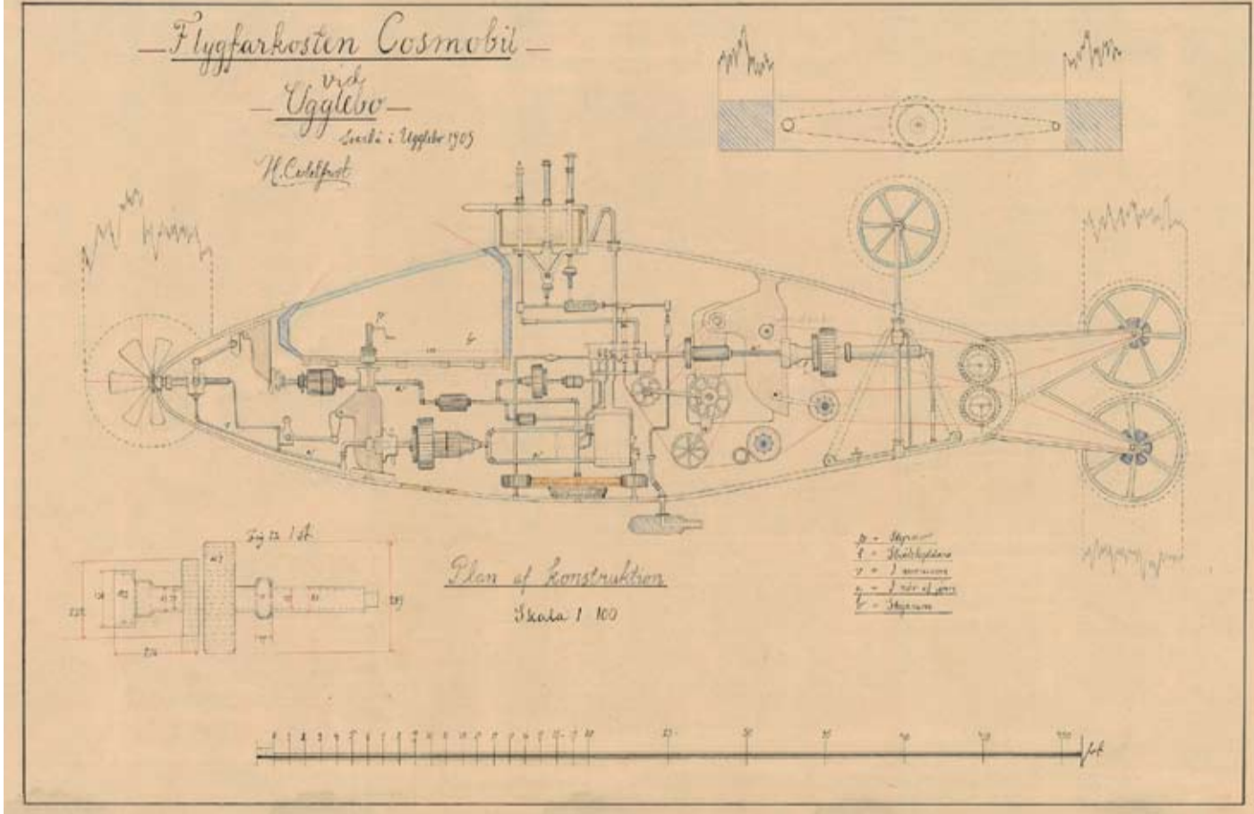
Ritning över Cosmobil av Ingenjör Henrik Cederfrost 1905
